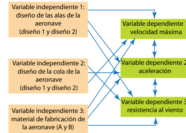
● Figura 8.22 Ejemplos de planteamientos gráficos o modelos en los que el modelo de análisis pertinente es el MANOVA (continuación).
