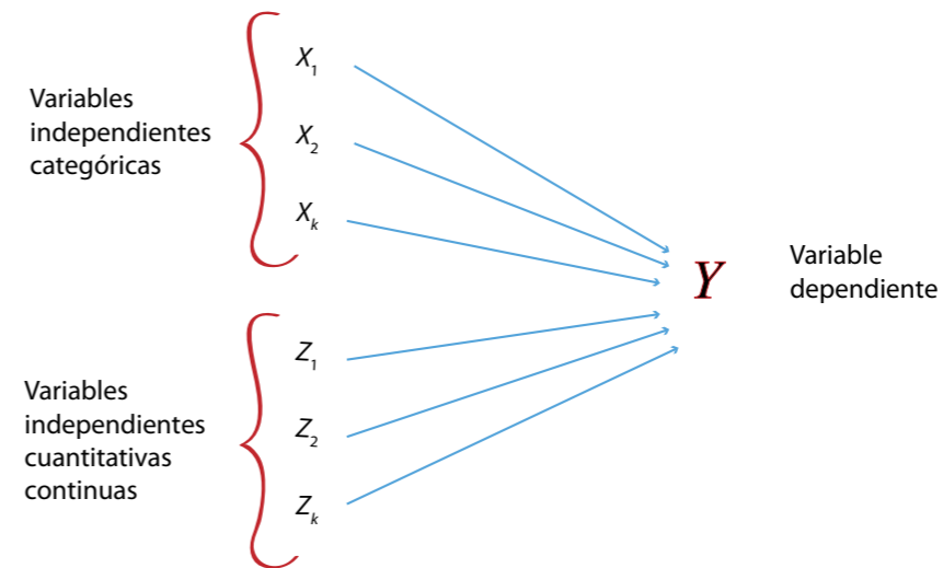
● Figura 8.7 Ejemplo de variables independientes que afectan a una dependiente.
