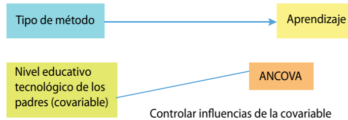
● Figura 8.12 Representación del control de la influencia de la covariable.
