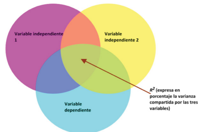
● Figura 8.18 Esquema de un coeficiente de determinación o correlación parcial.
