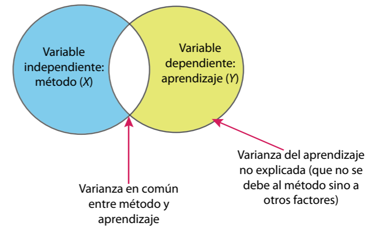
Figura 8.10 Representación a la varianza del aprendizaje debido al tipo de método y a otros factores.
