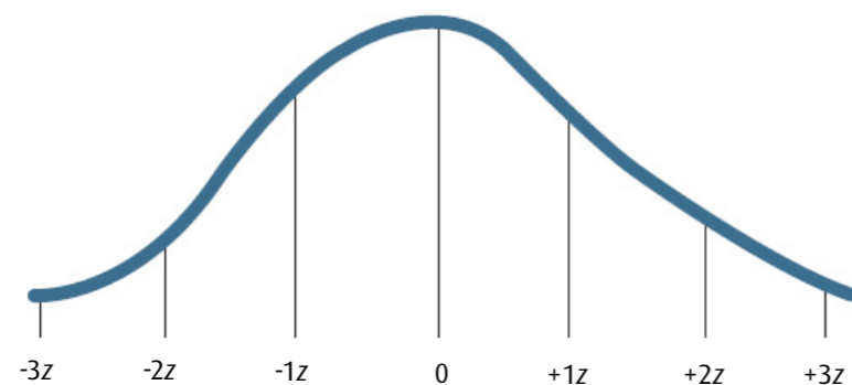
● Figura 8.1 Distribución de puntuaciones z .
