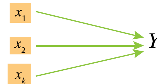
● Figura 8.6 Esquema de un análisis factorial de varianza.
