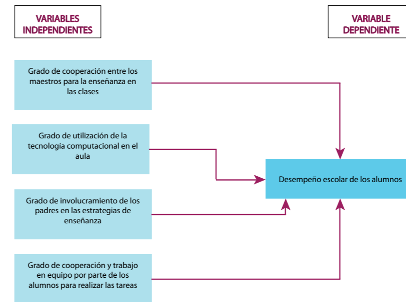
● Figura 8.17 Esquema de un modelo con una variable dependiente y varias independientes, en las que se pretende conocer el efecto de cada una de estas y los efectos conjuntos.
