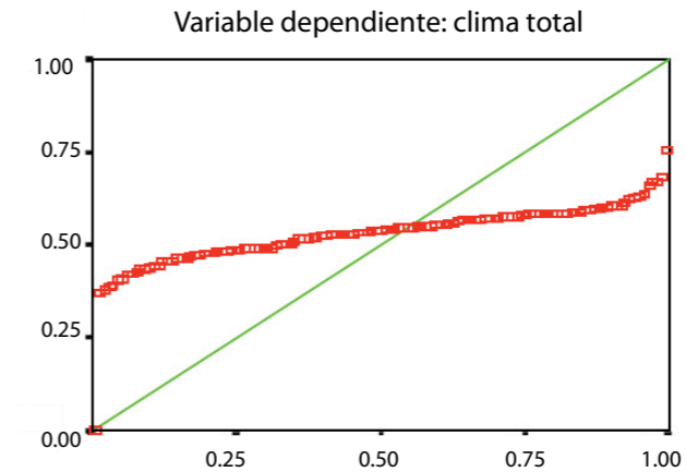
● Figura 8.21 Diagrama de dispersión del clima organizacional: laboratorio.
