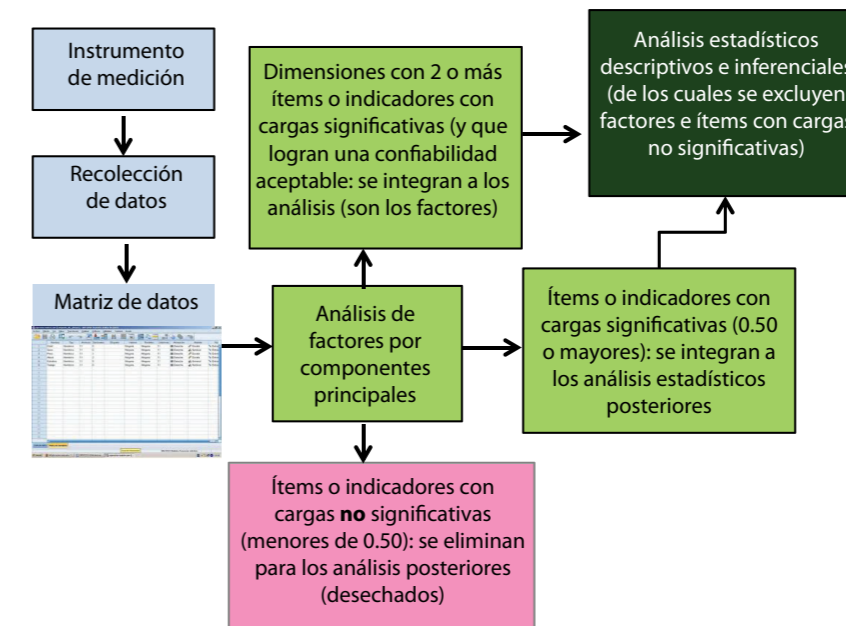
● Figura 8.16 Proceso para seleccionar ítems, reactivos o indicadores válidos de una medición a través del análisis de factores por componentes principales.
