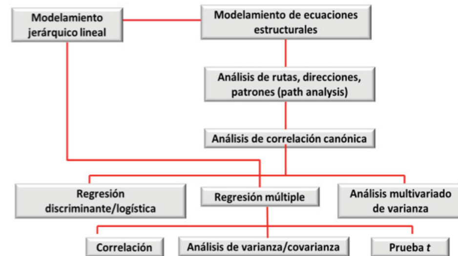
Figura 8.3 Familia del modelo lineal general de análisis.
